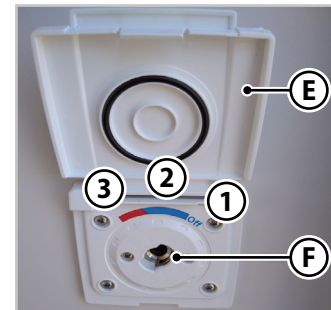
Sl.6.34 – Izhod za ročno prho
