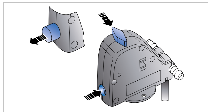
SI.6.40 – Varnostni ventil grelnika Combi
